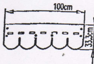
Bild 4: Befestigung
