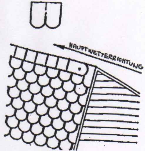
Bild 6: Dachfirst
