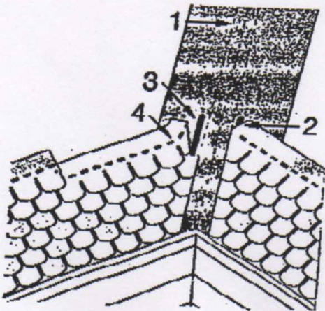
Bild 5: Kehle
