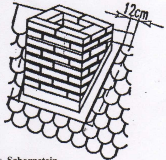
Bild 8: Schornstein
